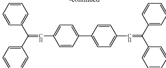
DPVBi
